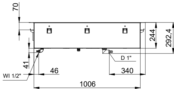
Oldalnézet
